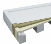
PRZEKRÓJ TECHNOLOGICZNY
